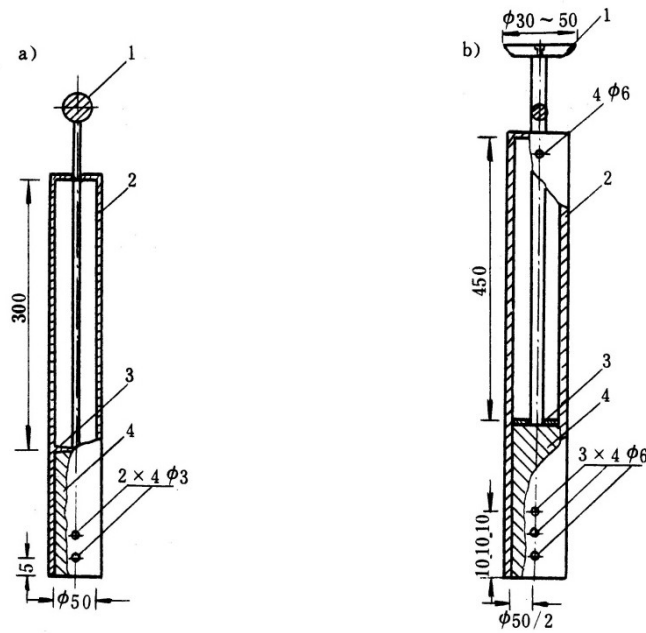
图 T0131-2 击锤和导杆 (单位: mm)
