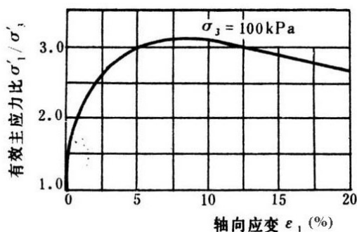
图 T0145-2 有效主应力比与轴向应变的关系曲线
