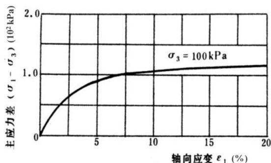
图 T0145-1 土应力差与轴向应变的关系曲线
